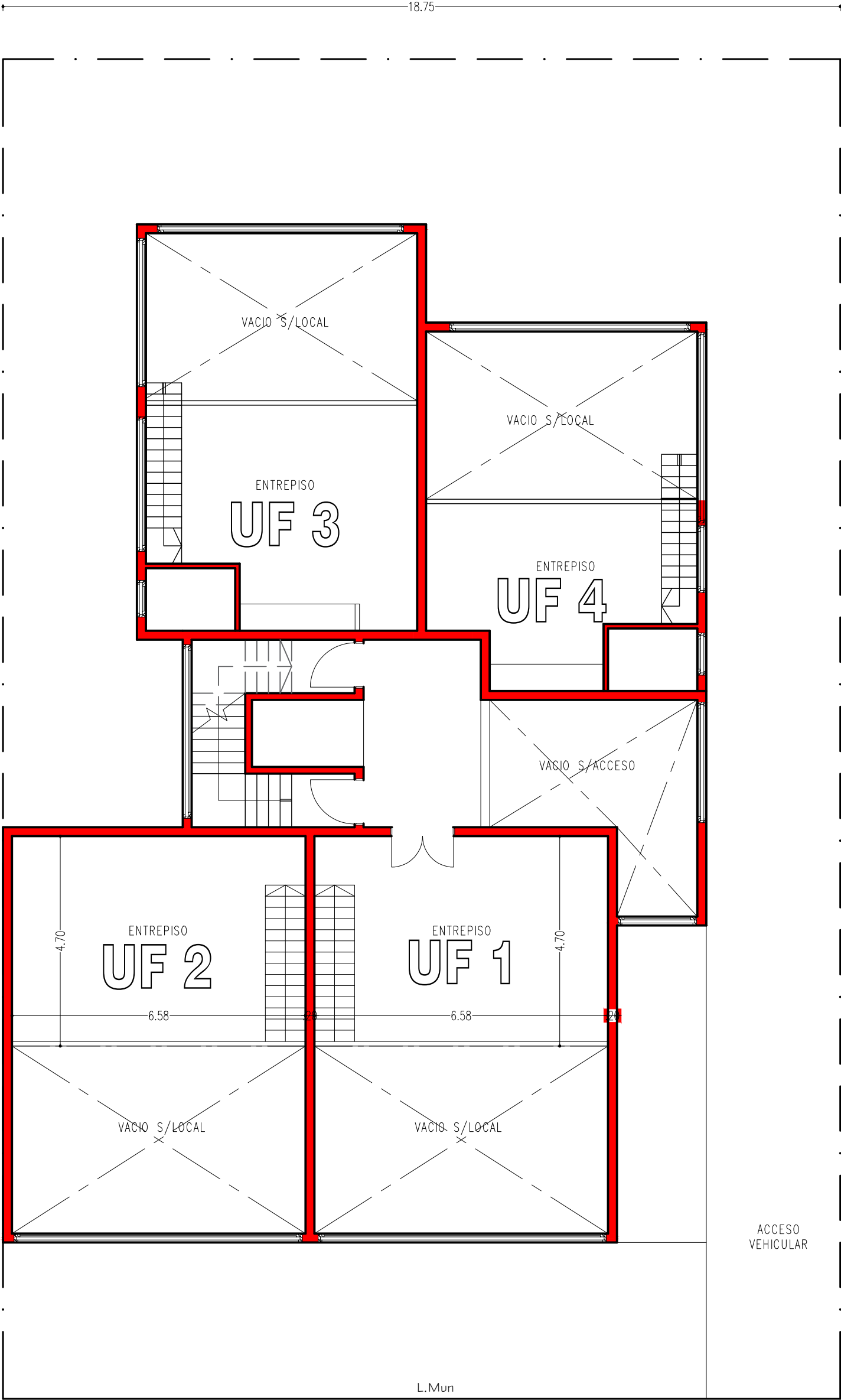
EJE CALLE DEL CANGREJO PLANTA ENTREPISO
